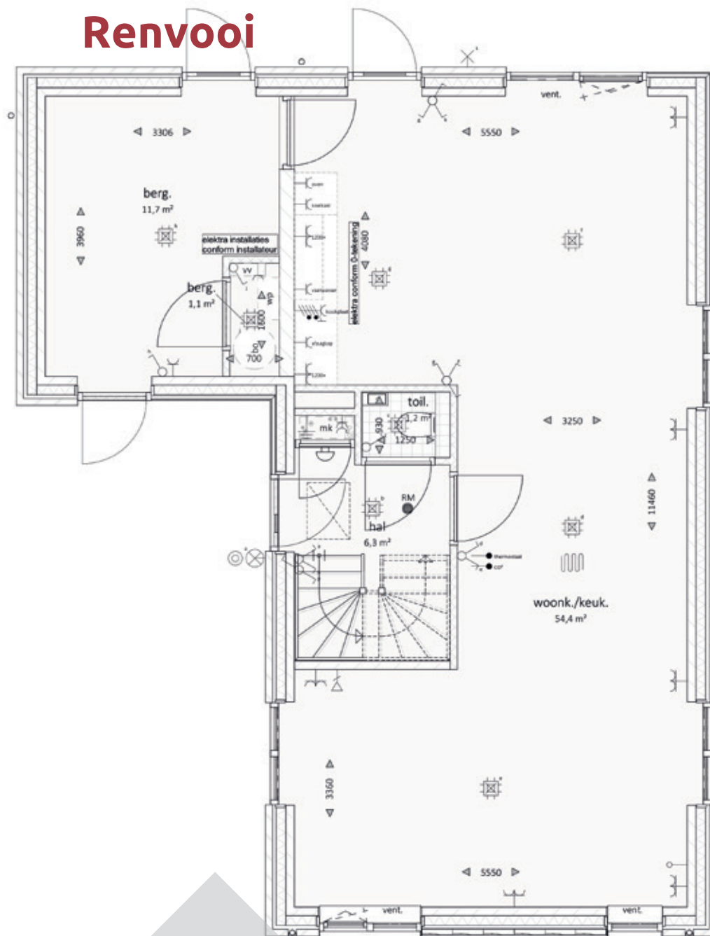
Begane Grond
