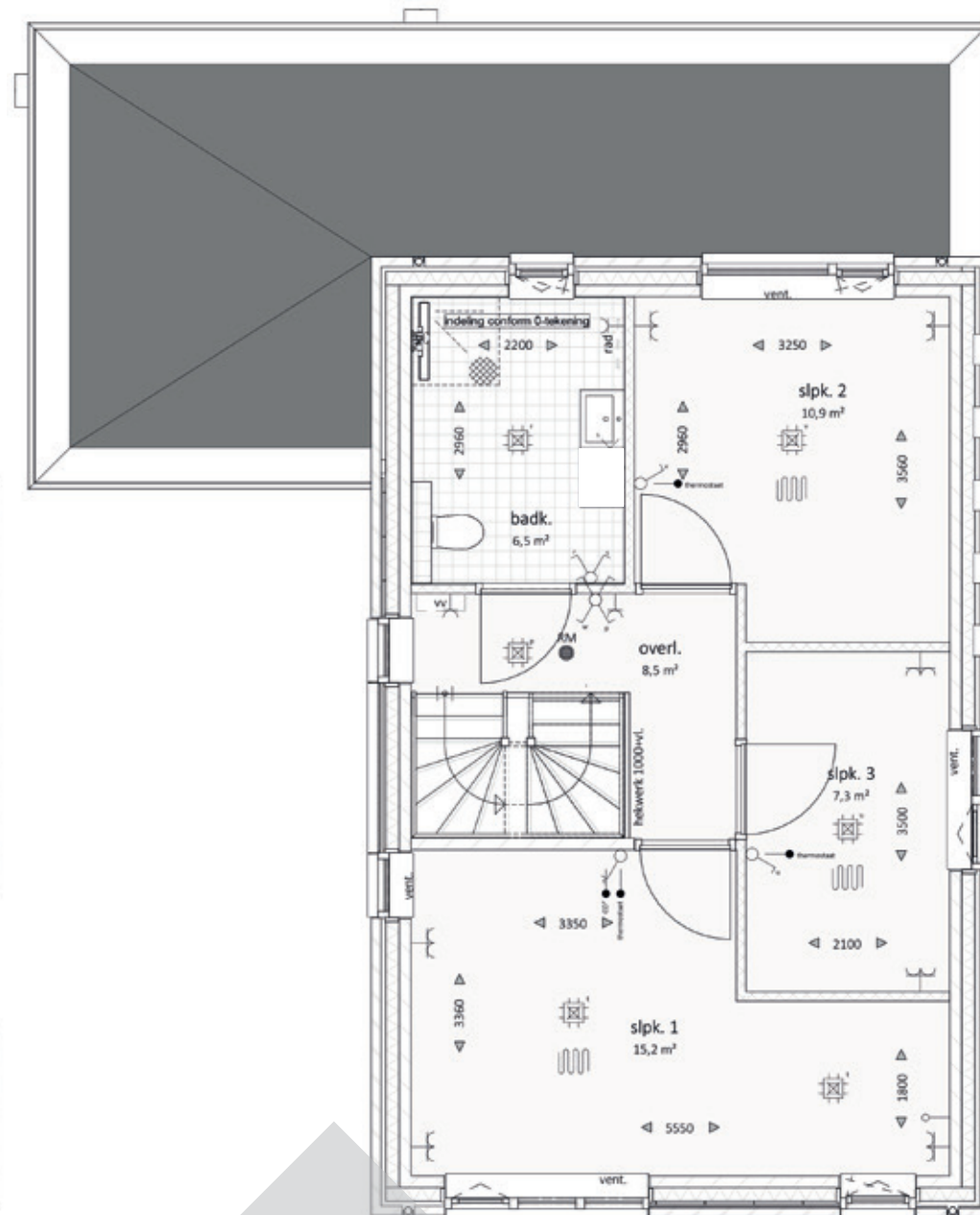
Eerste Verdieping
